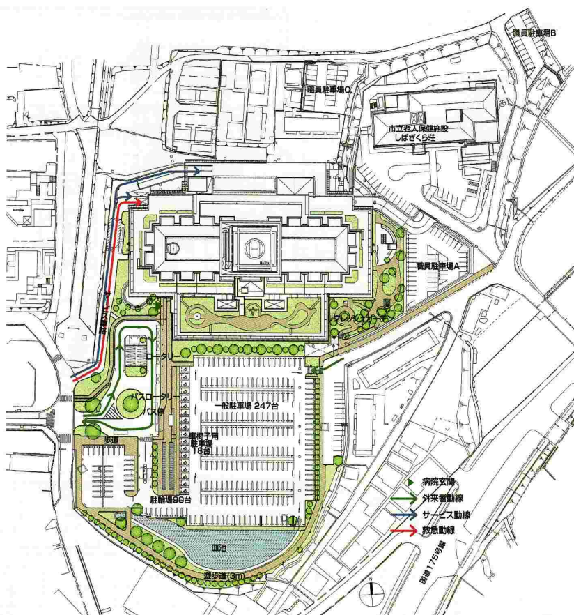
全体配置図 1/2,000
